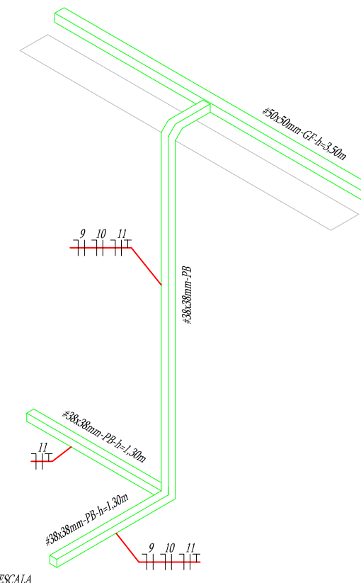
SEM ESCALA DETALHAMENTO DAS DESCIDAS DE PERFILADO PARA TOMADAS DE COMPUTADORES NOS LABORATÓRIOS
