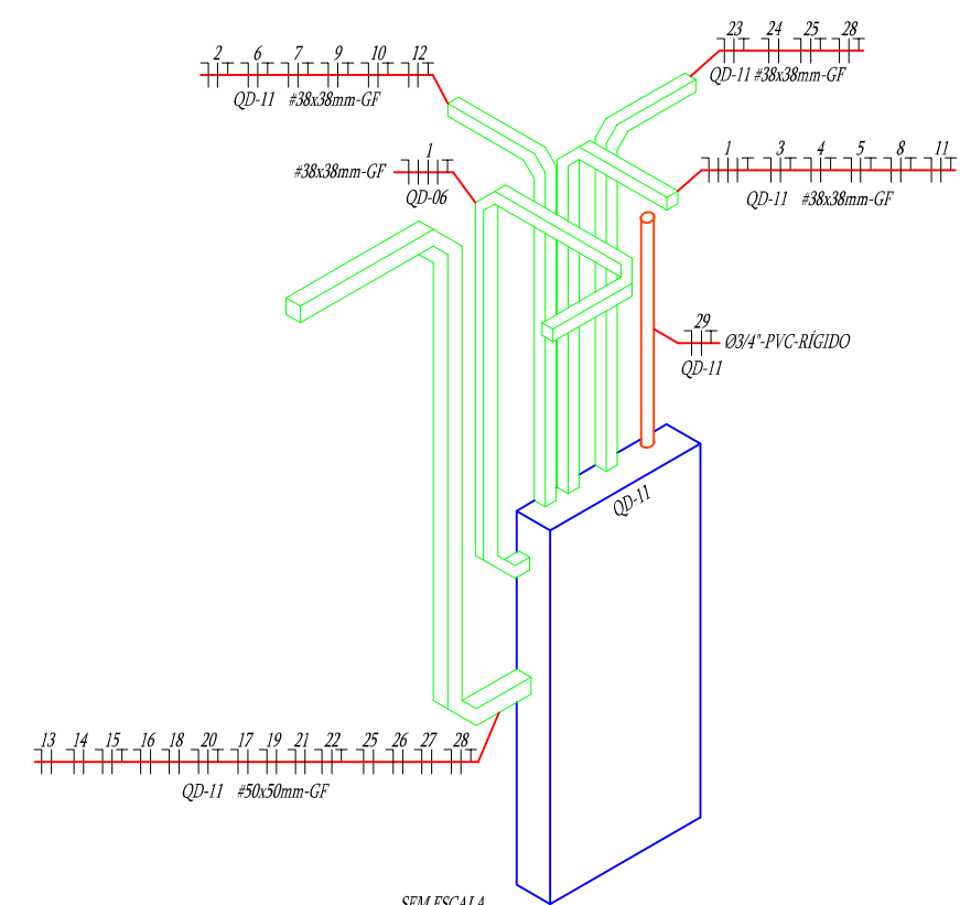
SEM ESCALA DETALHAMENTO DAS SAÍDAS DE ELETRODUTOS E PERFILADOS DO QUADRO DE DISTRIBUIÇÃO QD-11
