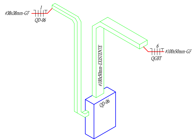
SEM ESCALA DETALHAMENTO DAS SAÍDAS DE ELETRODUTOS E PERFILADOS DO QUADRO DE DISTRIBUIÇÃO QD-06
