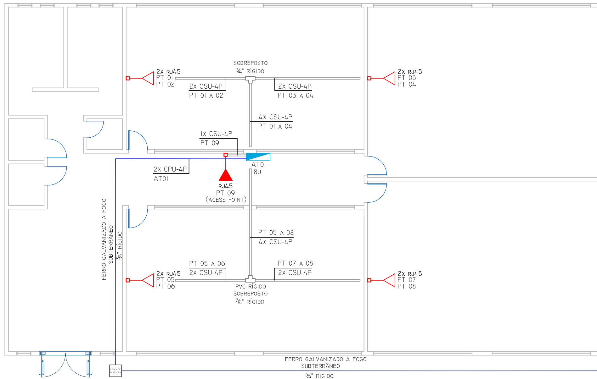
01 PLANTA BAIXA ESCALA 1:100
