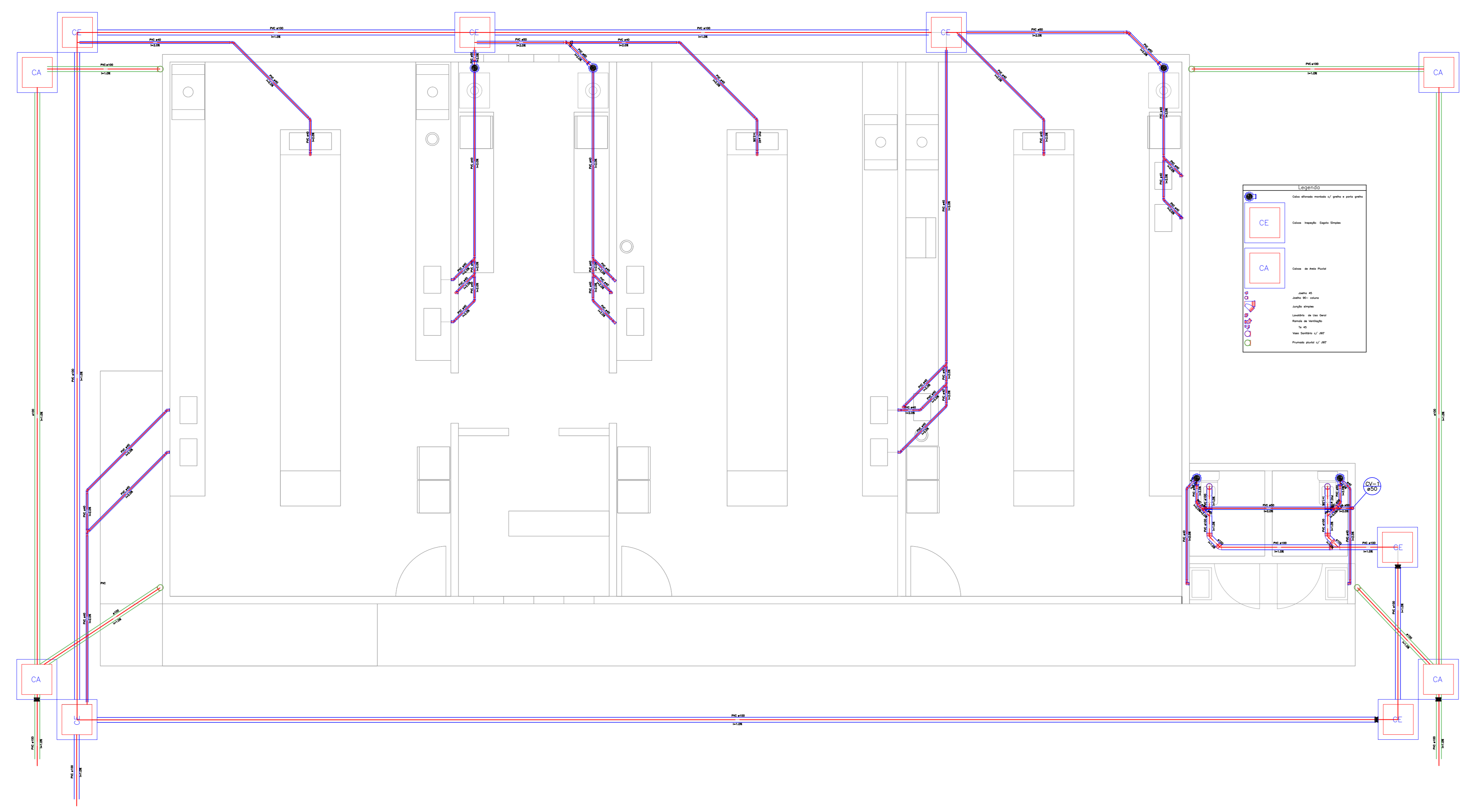
2 INSTALAÇÕES SANITÁRIAS E PLUVIAIS ESCALA 1:50
