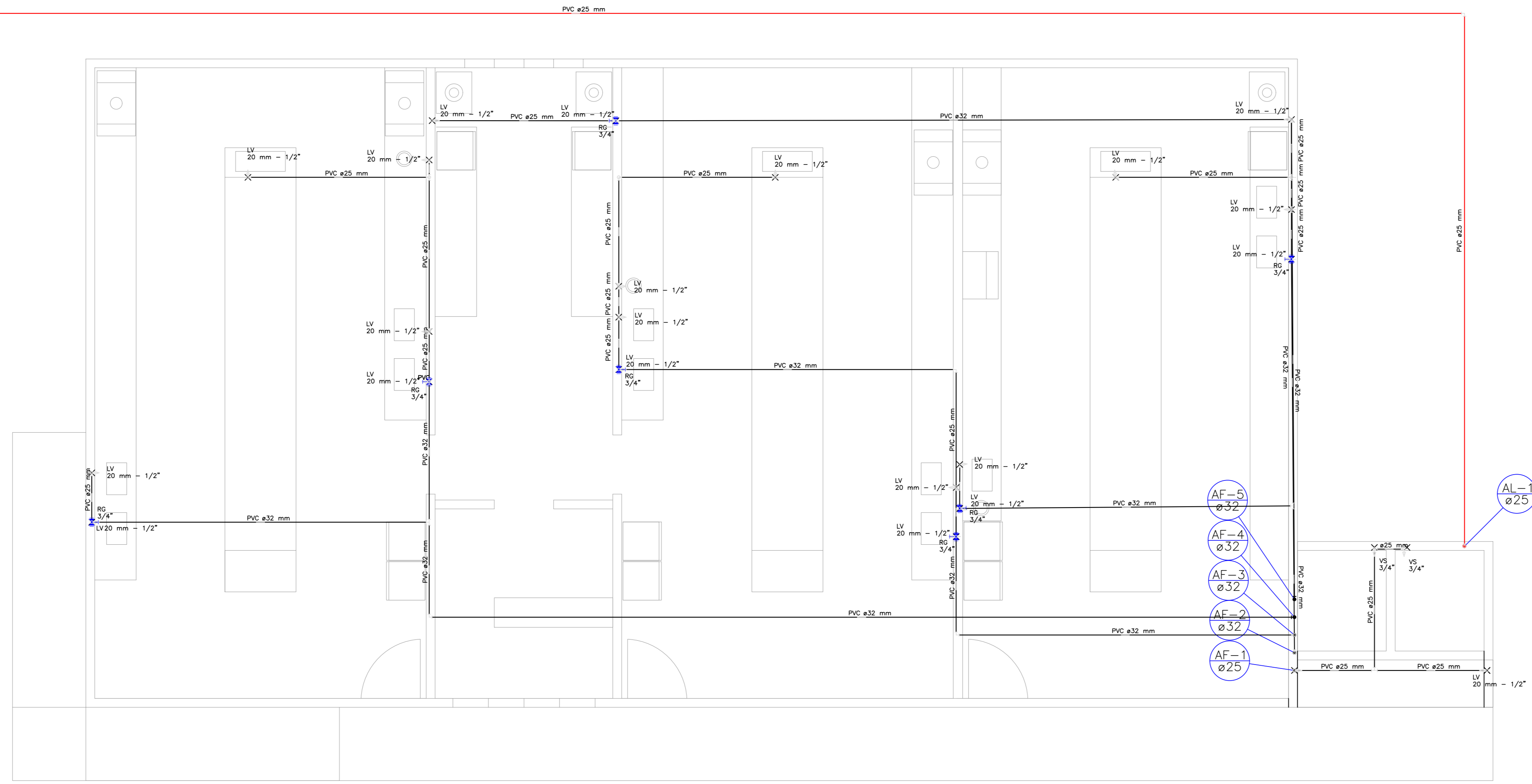
1 INSTALAÇÕES HIDRÁULICAS PAV. TÉRREO ESCALA 1:50
