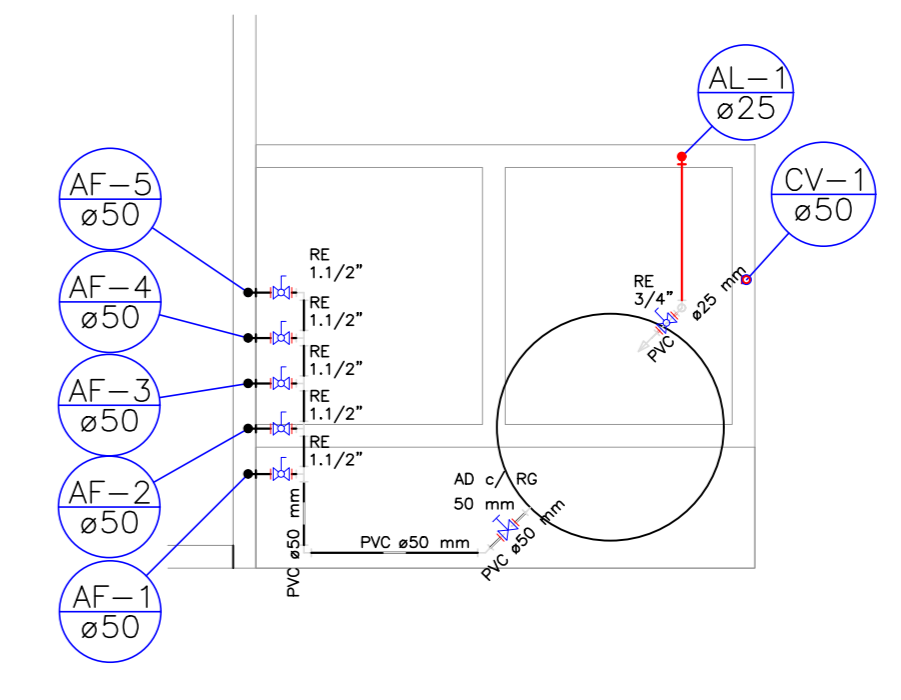
3 INSTALAÇÕES HIDRÁULICAS RESERVATÓRIO ESCALA 1:50
