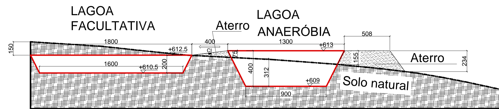
CORTE AA Escala 1:20
