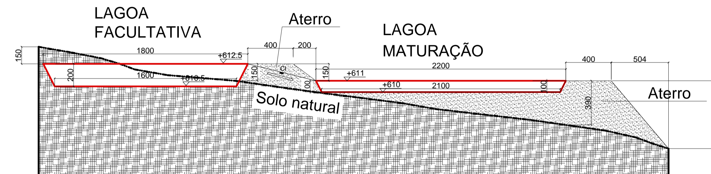
CORTE BB Escala 1:20
