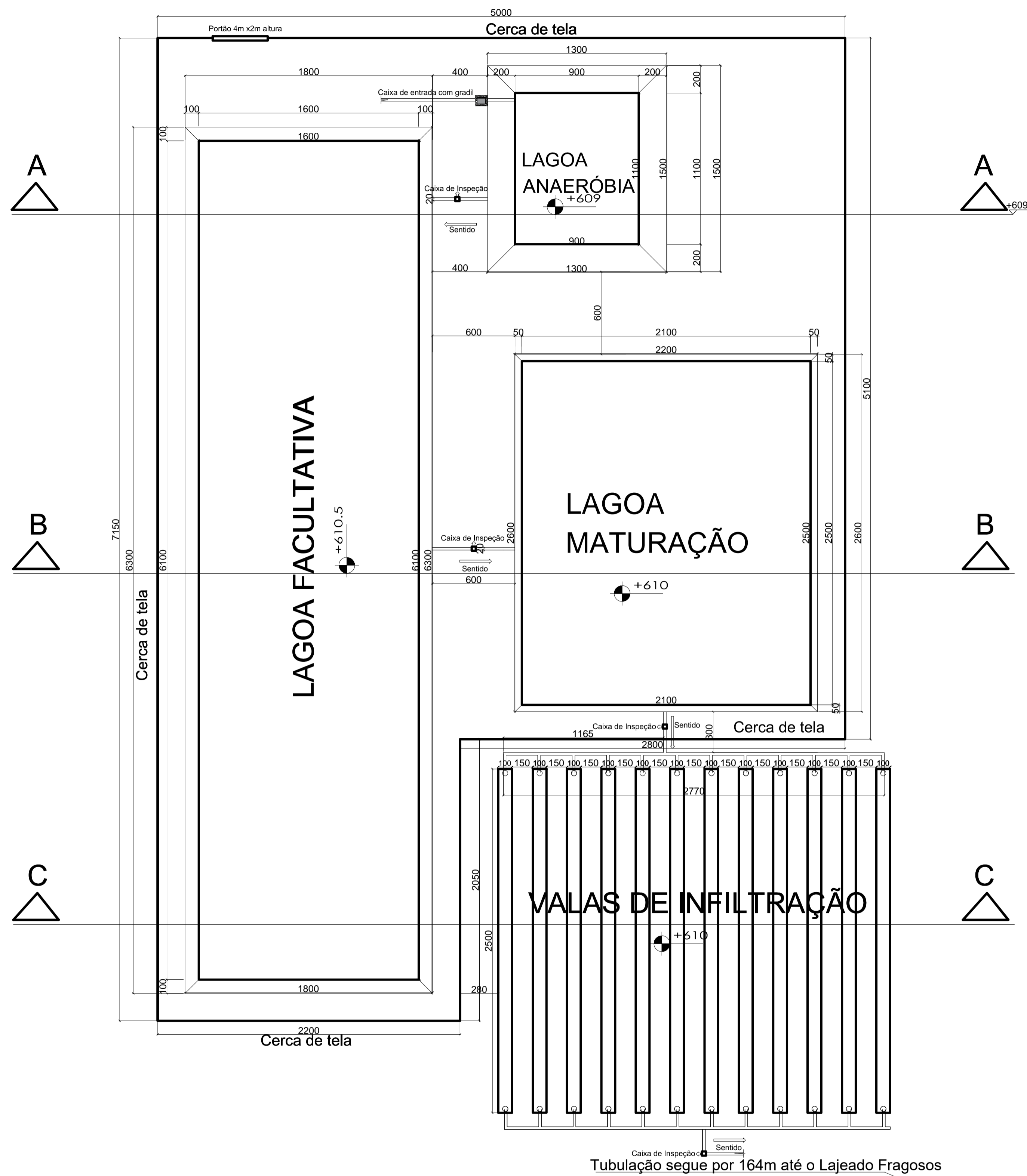
PLANTA BAIXA SISTEMA DE TRATAMENTO DE ESGOTO ESCALA 1:20
