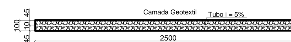
DETALHE DA VALA DE INFILTRAÇÃO Escala 1:20
